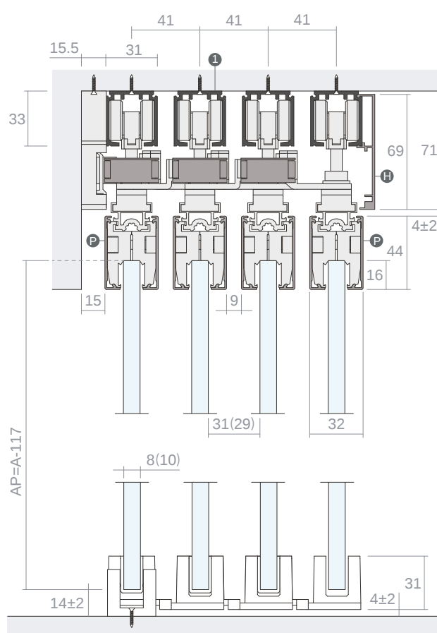
APLICAÇÃO NA PAREDE - MÁX. 4 PORTAS
