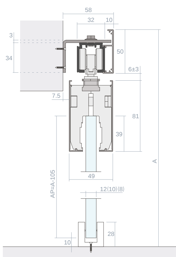
PORTA COM FIXAÇÃO NA PAREDE
