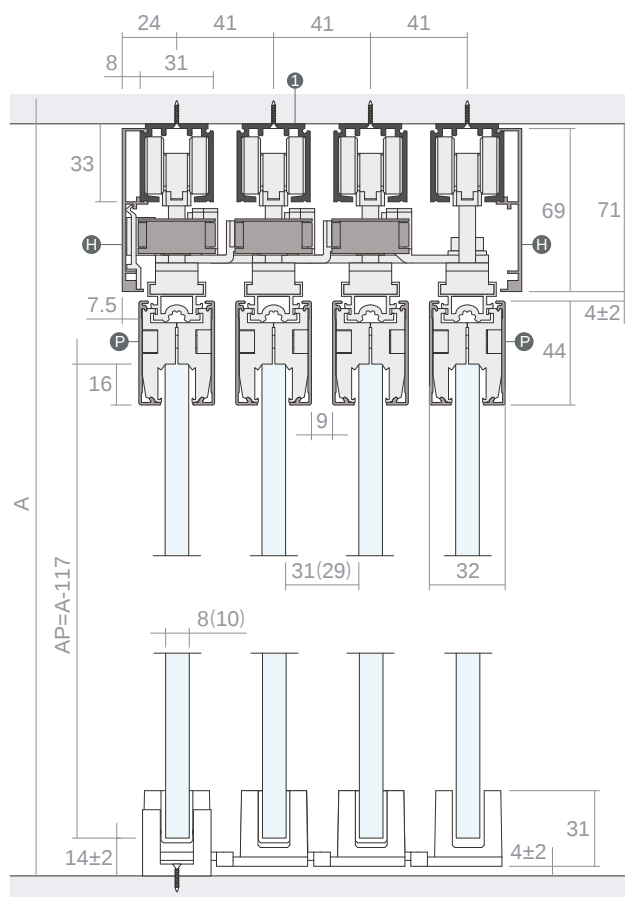
APLICAÇÃO AO TETO - MÁX. 4 PORTAS
