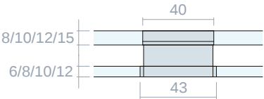
DETALHE PARA FURO PARA VIDRO TEMPERADO COM CAMARA M14
