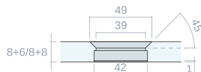
DETALHE PARA FURO PARA VIDRO LAMINADO M14
